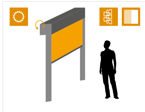
Basisausführung bei zipSCREEN.2, PURO 2.XR-zip mit Führungsschiene 33x61 mm und rollSCREEN.2
