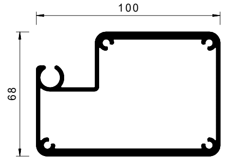
Fallstange mit integrierter Wasserablafrinne
