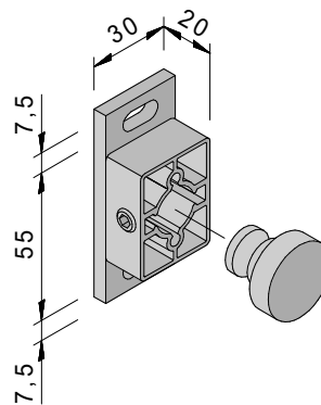
Führungsschienenhalter (optional)
