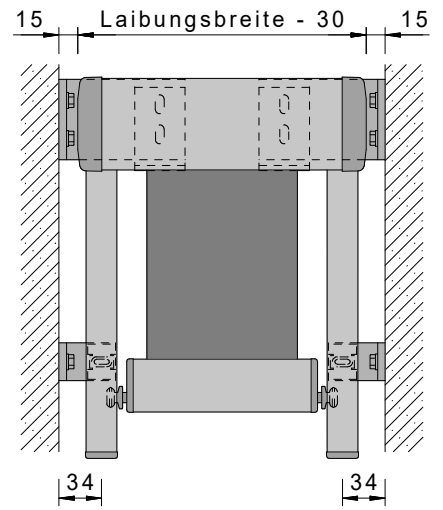
Laibungswinkel Schiene
