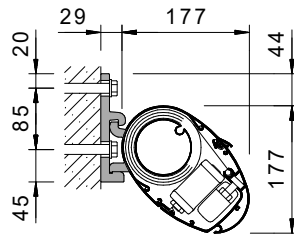
Wandmontage maximale Neigung
