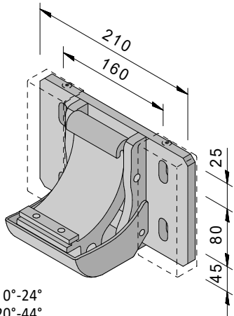
Distanz-Wandkonsole
