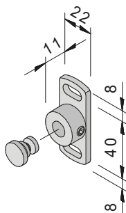
Führungsschienenhalter
