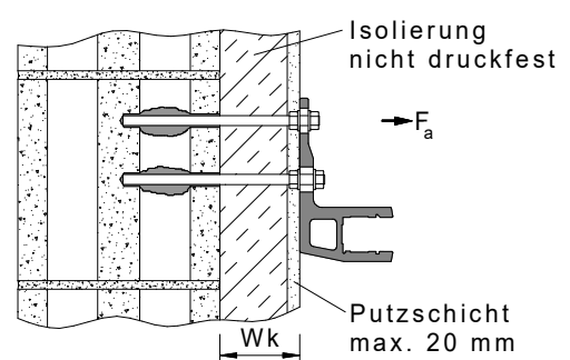
Montagebild 16
