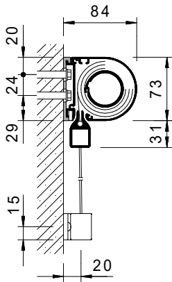
Seilspanner Wand
