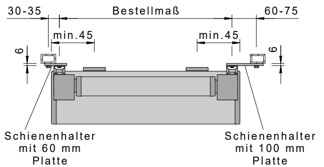
Montage mit versetzter Platte
