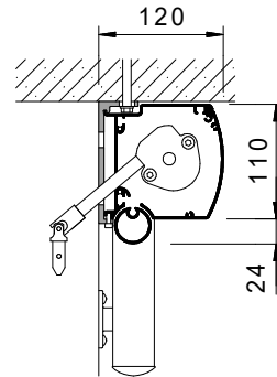
Getriebeabgang, schräg hinten (F412, Option)
