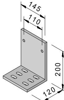
Dachsparrenhalter gerade
