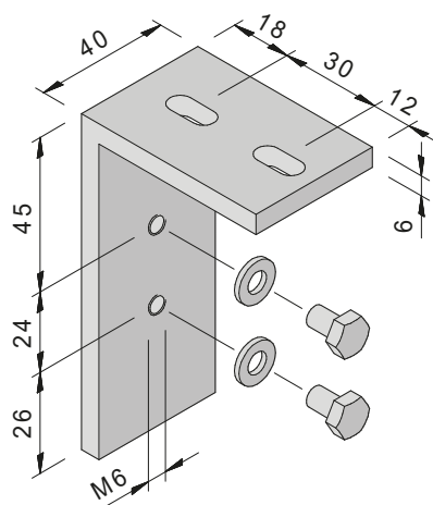
Deckenwinkel für Wandkonsole
