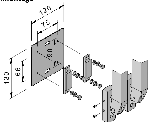
Reihenmontage
