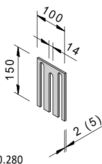
Futterstück Deckenmontage
