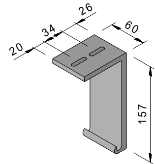
Deckenkonsole +100 mm für Führungsschienehalter 130 mm
