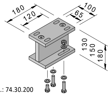
Distanzhalter für Deckenmontage
