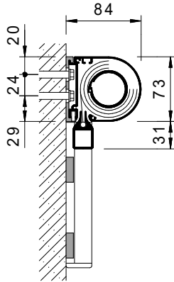
Führungsschiene
