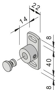
Führungsschienehalter
