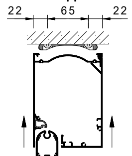
Deckenmontage, Kasten einklippsen
