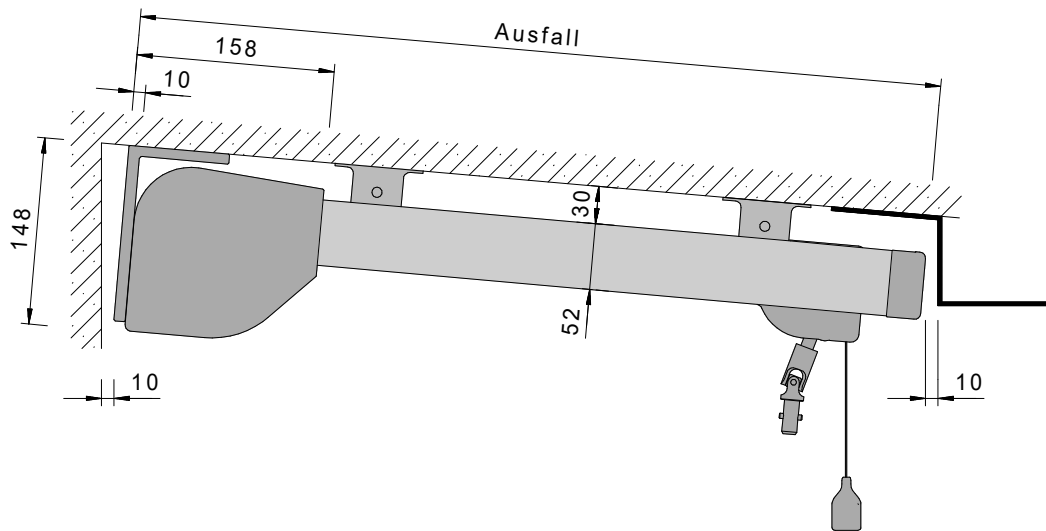
Fallprofil
