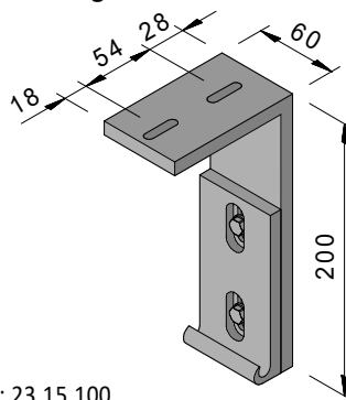
Deckenkonsole +50 mm für Führungsschienehalter 80 mm
