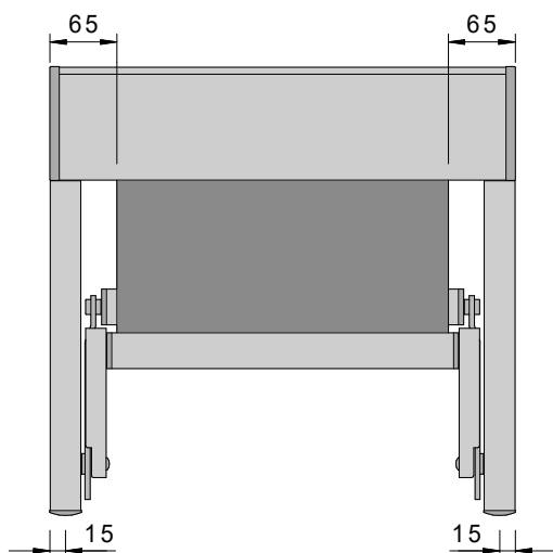
einteilig, Vorderansicht
