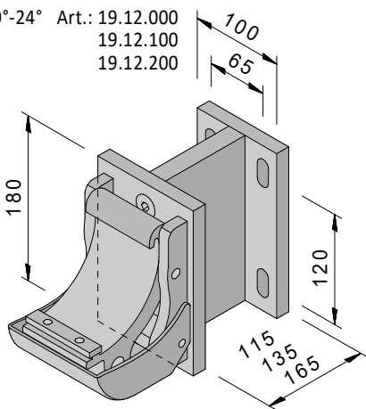
Distanz-Wandkonsole
