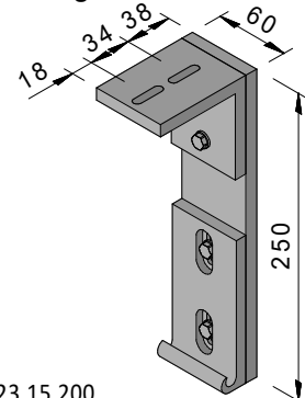
Deckenkonsole +100 mm für Führungsschienehalter 130 mm
