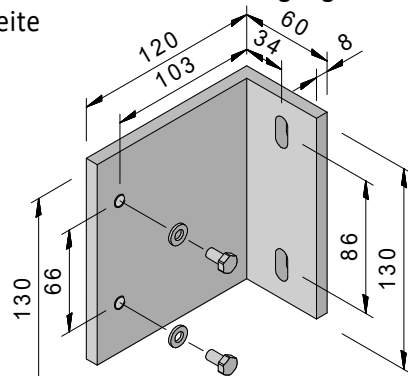
Reihenmontage
