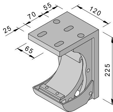
Deckenkonsole (0-24°) 120 mm
