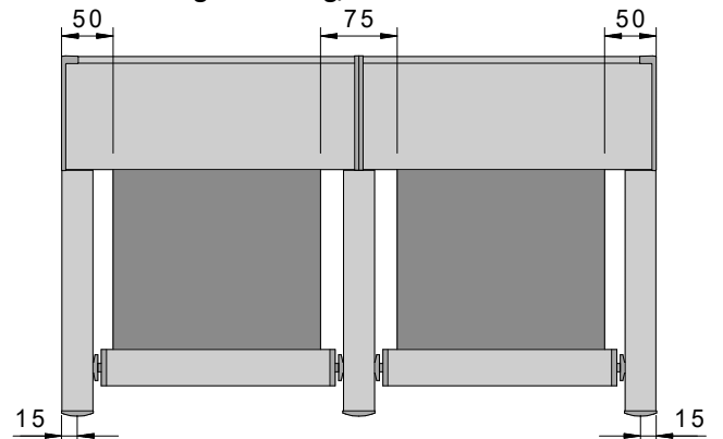
Schienenführung zweiteilig, Vorderansicht
