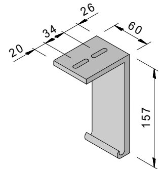
Deckenkonsole +100 mm für Führungsschienenhalter 130 mm
