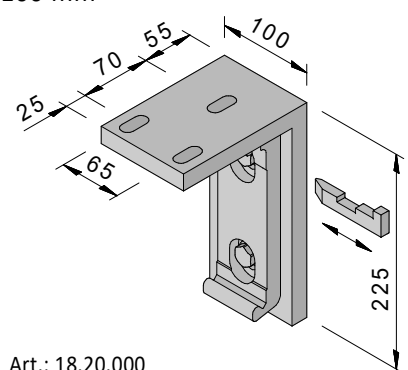
Deckenwinkel 100 mm
