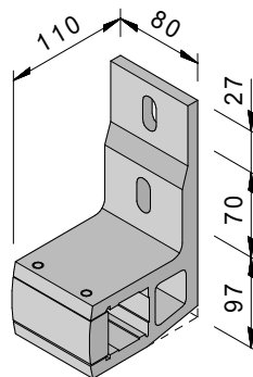
Wandkonsole 80 mm
