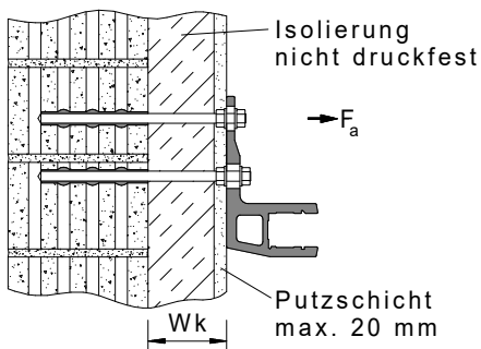
Montagebild 15
