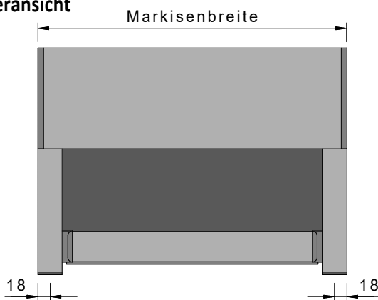
Abdeckprofil
