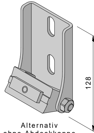
Absenkbare Schienenstütze (optional)
