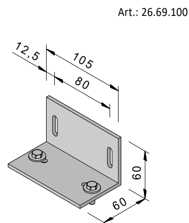
Laibungswinkel für Schienenhalter (bevel angle for rail holder)
