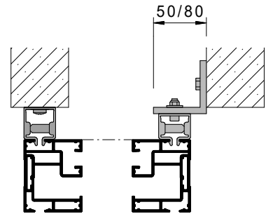
Befestigung mit Winkel
