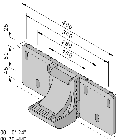
Deckenkonsole (20-44°) 120 mm
