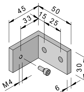
Laibungswinkel Schiene
