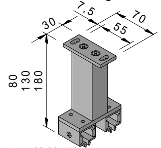
Verlängerter Doppel-Führungsschienehalter für gekuppelte Anlage für Reihenmontage
