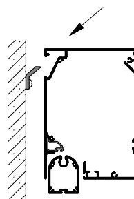
Wandmontage, Kasten einklippsen
