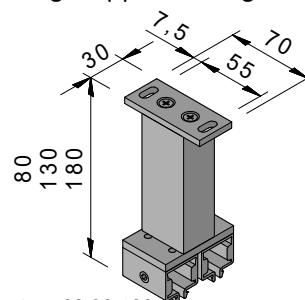
Verlängerter Doppel-Führungsschienehalter für gekuppelte Anlage für Reihenmontage
