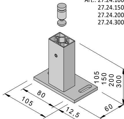
Schienenhalter für 1/2 Reihenmontage
