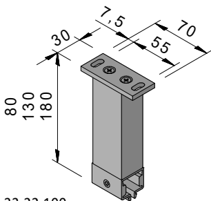
Verlängerter Führungsschienehalter
