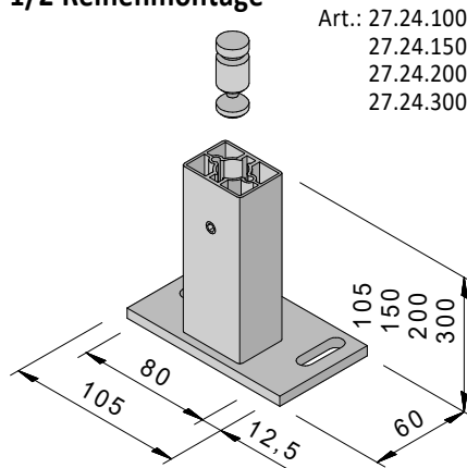
Schienenhalter 300 mm nicht für Version mit Zip
