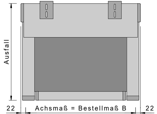
Draufsicht einteilig
