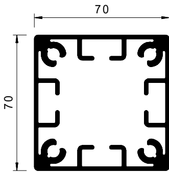
Standard-Schienenstütze / Quertraverse
