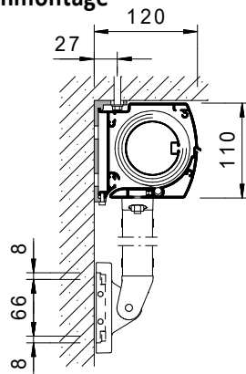
Laibungswinkel für Universalkonsole
