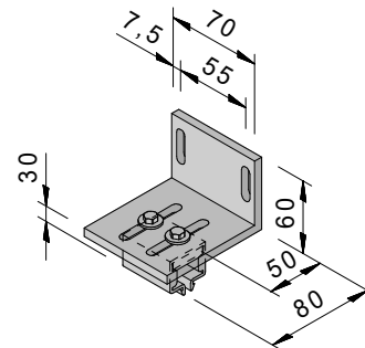
Laibungswinkel GetriebeSeite mit Führungsschienenhalter
