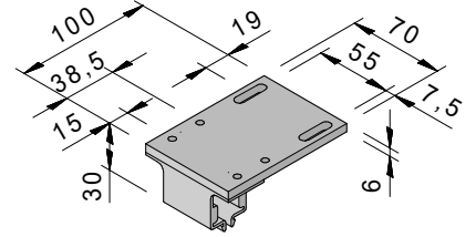
Montageplatte für eingerückte Montage mit Führungsschienenhalter
