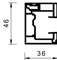
Führungsschiene klein (Standard)
