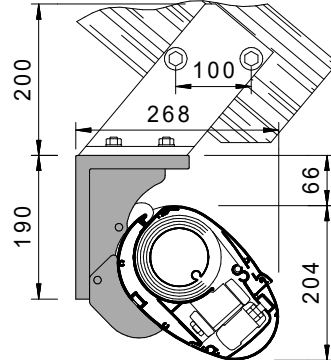
Dachsparrenmontage schräger Halter, maximale Neigung
