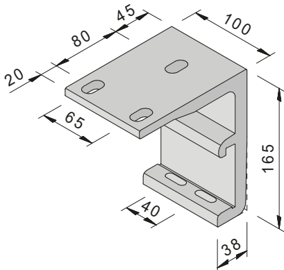
Deckenkonsole 100 mm
