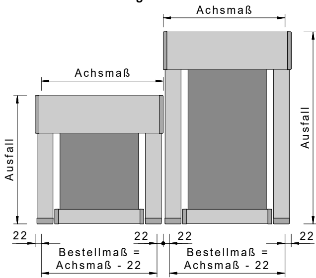
Führungsschiene
