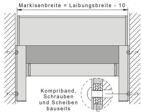
Montage durch die Schiene
