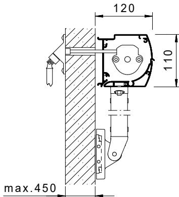
Wandmontage Innenbedienung mit Knickkurbel
