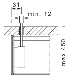
Innenbedienung, Draufsicht
