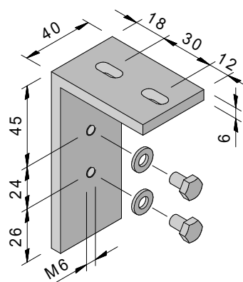
Deckenwinkel für Wandkonsole
