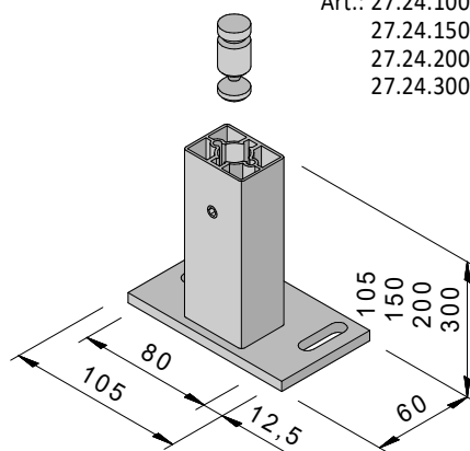
Schienenhalter für 1/2 Reihenmontage (rail holder for 1/2 row mounting)
