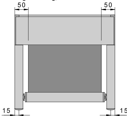
Schienenführung einteilig, Vorderansicht
