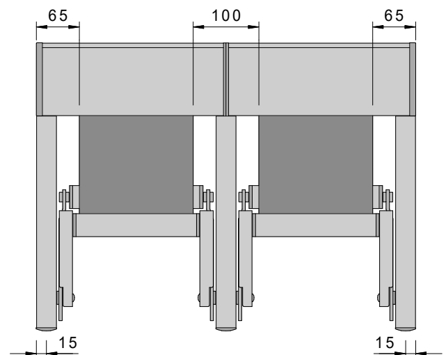
zweiteilig, Vorderansicht
