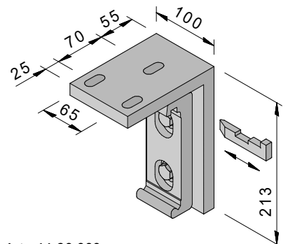
Deckenwinkel 100 mm
