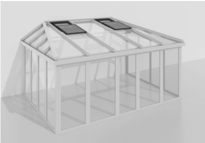
Hebe-Schiebefenster Motorisches Öffnen und Schließen. Sehr flach, sodass z. B. der Betrieb einer Markise nicht gestört wird.
